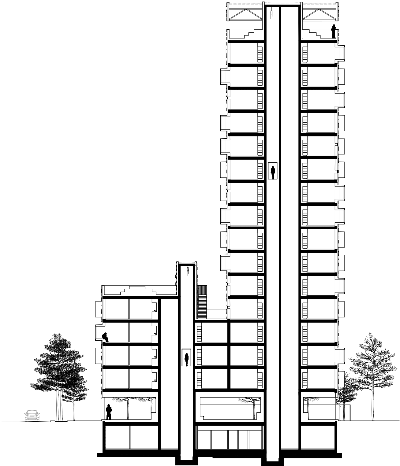
LÆNGDESNIIT 1:300
