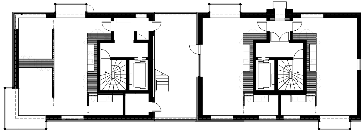
ETAGE 04 1:200
