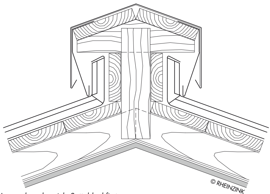
Anwendungsbereich: Satteldachfirst Ausführungsvariante: hohe Ausführung mit Quetschfalz
