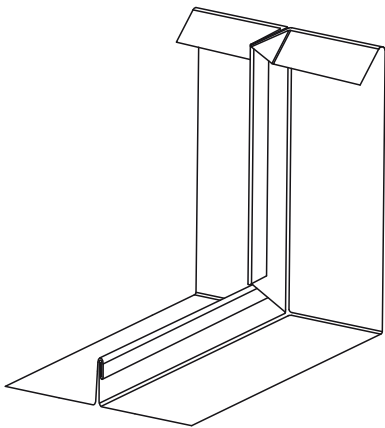
Schulungsbauteil: Quetschfalz an aufgehendes Bauteil
