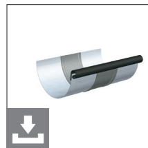
Bewegungsausgleicher, halbrund, walzblank, Bewegungsteil zinkgrau, Wulstkappe basalte, 260 mm Länge
