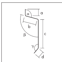
Kaplleiste, glatt, 3 m Länge
