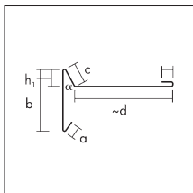
Windbordleiste, Falz, 3 m Länge
