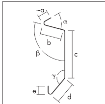
Kapelleiste, Falz für Abdichtung, 3 m Länge
