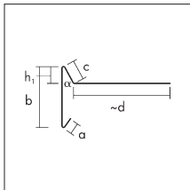
Windbordleiste, glatt, 3 m Länge
