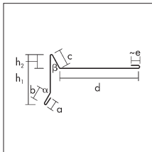
Windfeder, Falz, 3 m Länge
