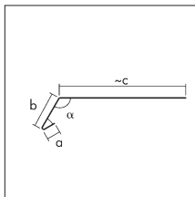
Taufstreifen, glatt, 105°, 3 m Länge
