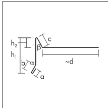
Windfeder, glatt, 3 m Länge
