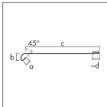
Taufstreifen, Falz, mit Wulst, 3 m Länge
