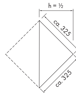
Sichtfläche – Rastemaße
