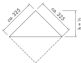
Sichtfläche – Rastemaße
