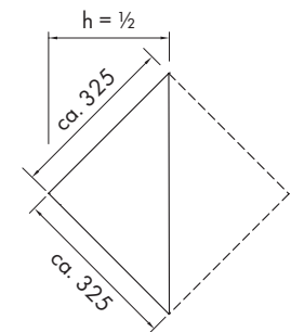
Sichtfläche – Rastemaße
